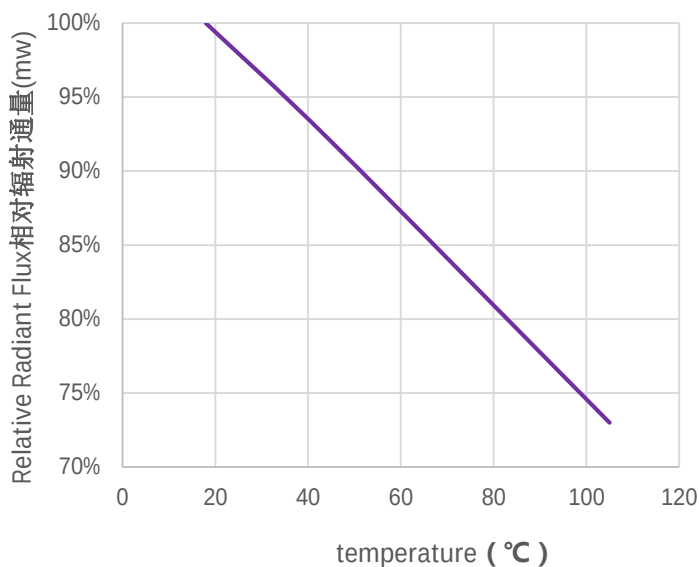
(4) 相对辐射通量与结温的关系 RELATIVE LUMINOUS Intensity VS. TEMPERATURE
